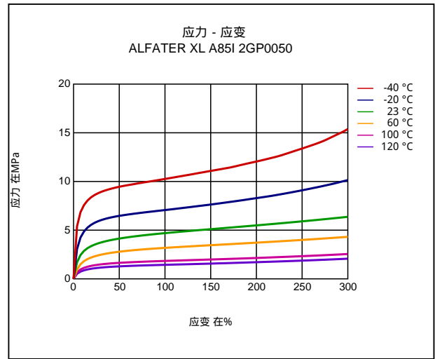
应力 - 应变
